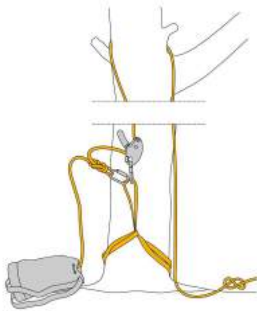
Fig. 8 - Ancoraggio svincolabile della fune alla base dell'albero
